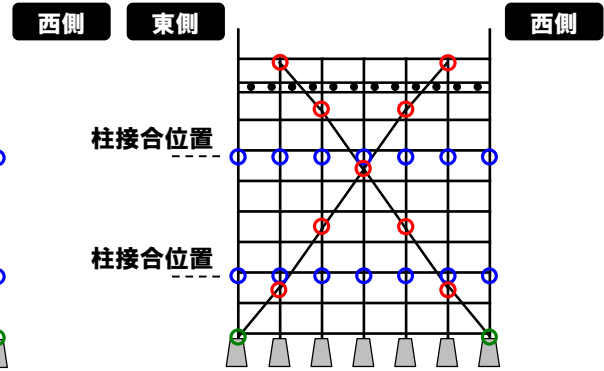
Main Bent (東-西)
