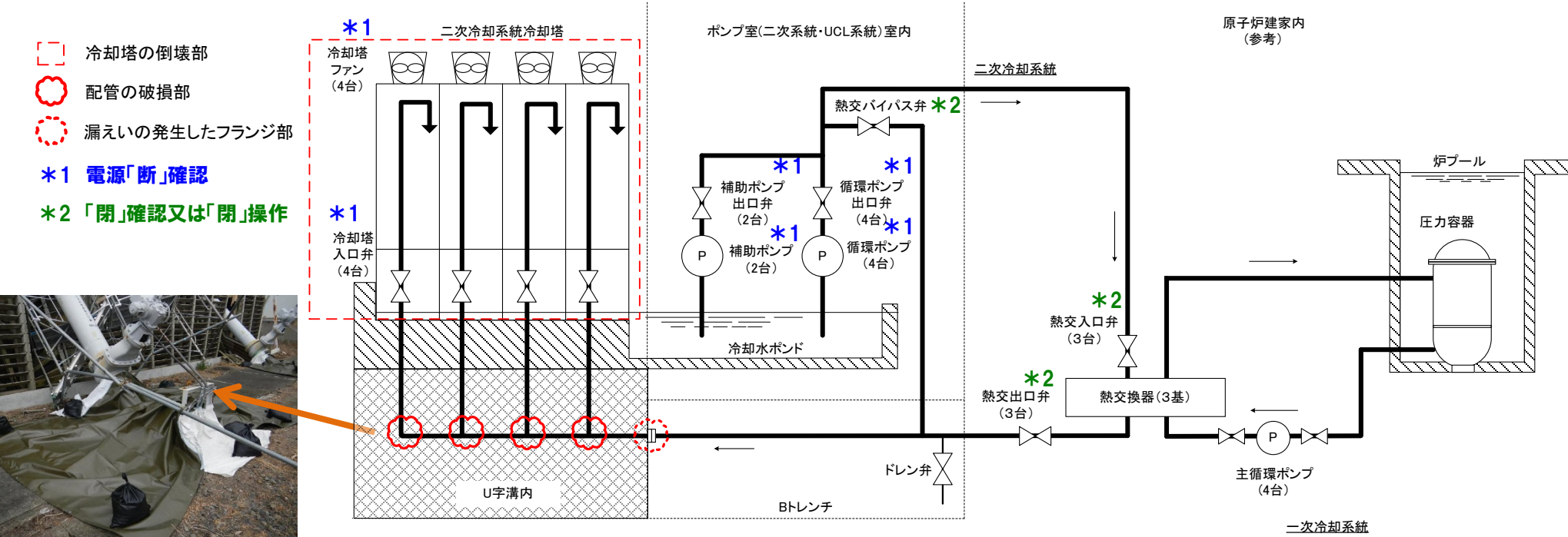
二次冷却系配管の養生
