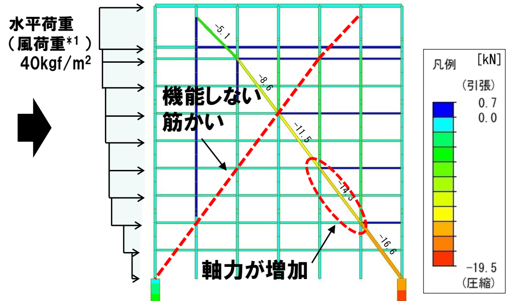
(2) 木材の腐朽により機能しない場合
