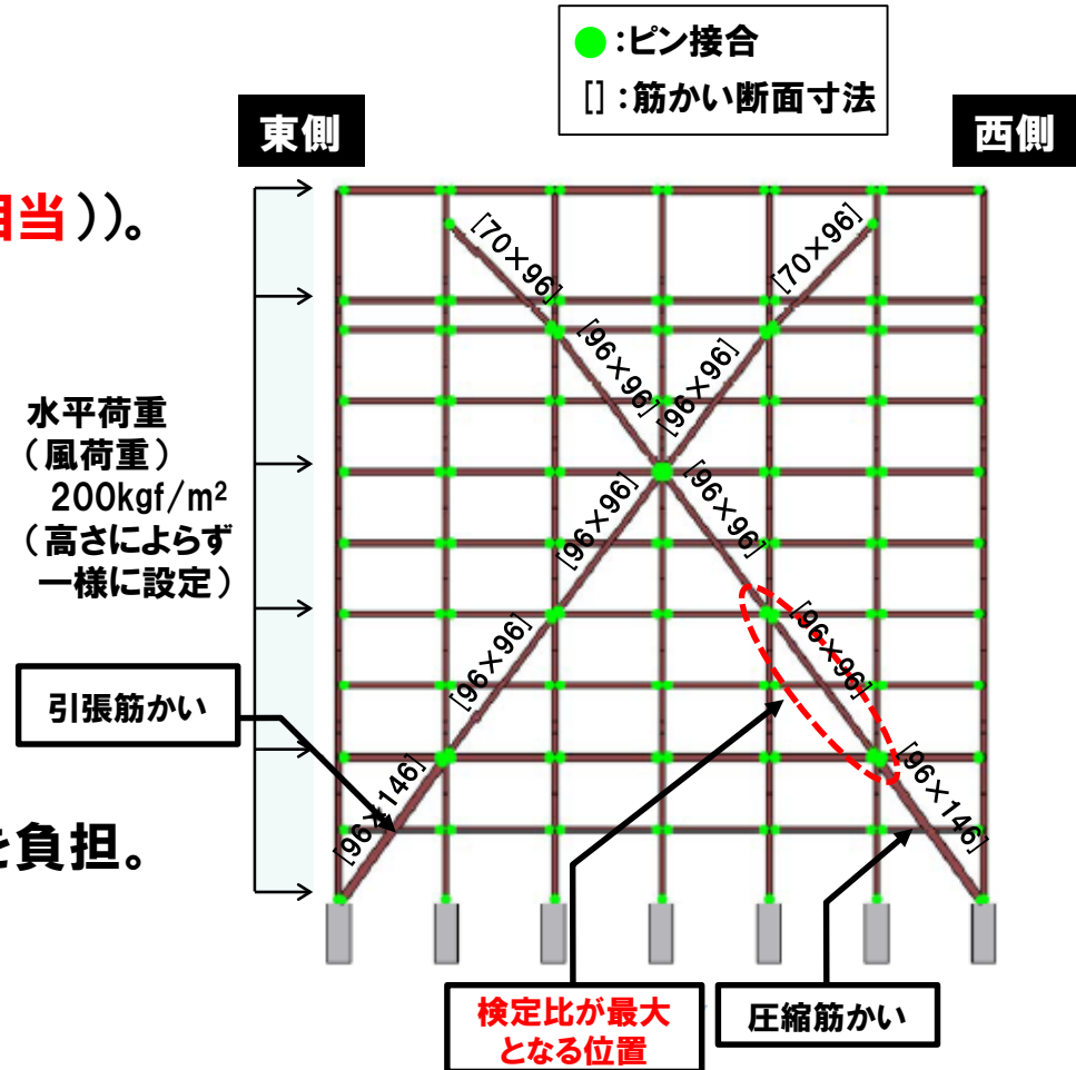
冷却塔東西断面のモデル化(例)
