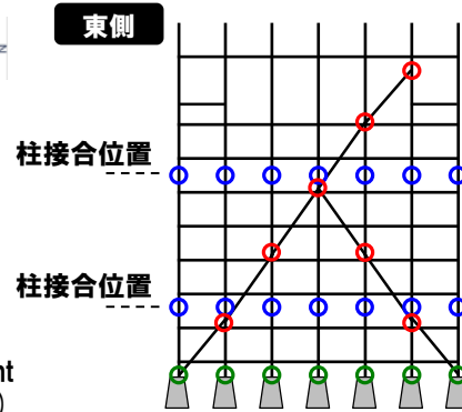
Part'n Bent (東-西)
